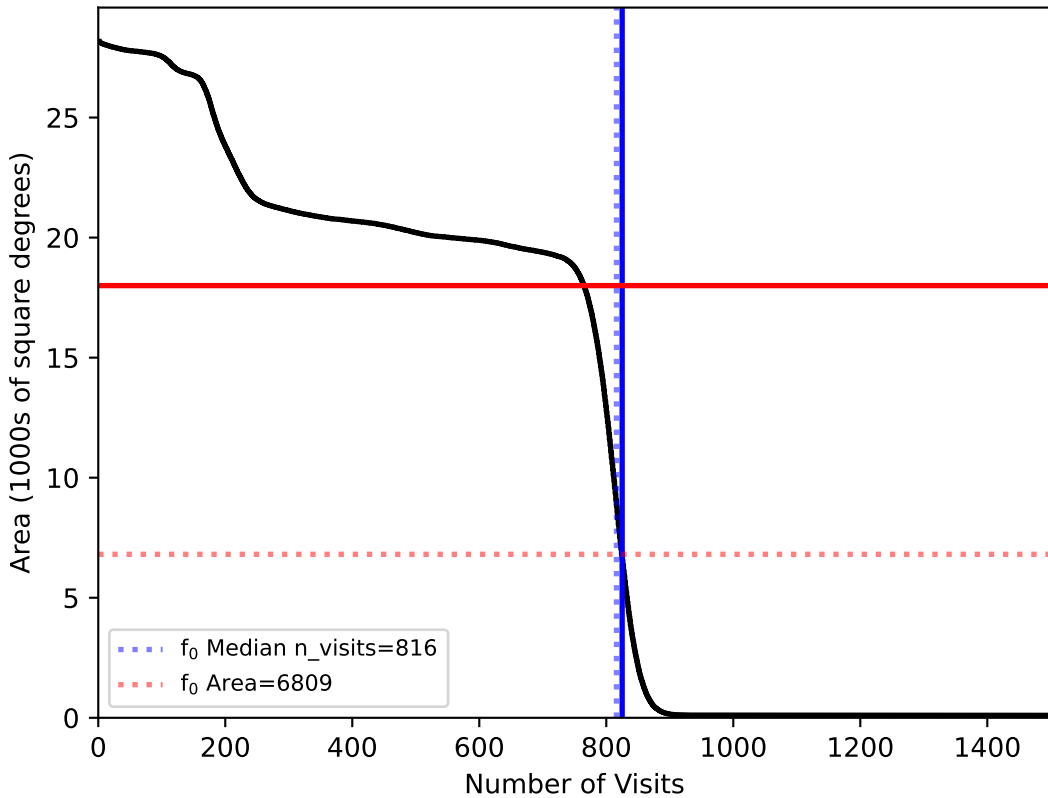
too_elab_r16_d2_ugrizy_v3.4_10yrs All sky: f0
