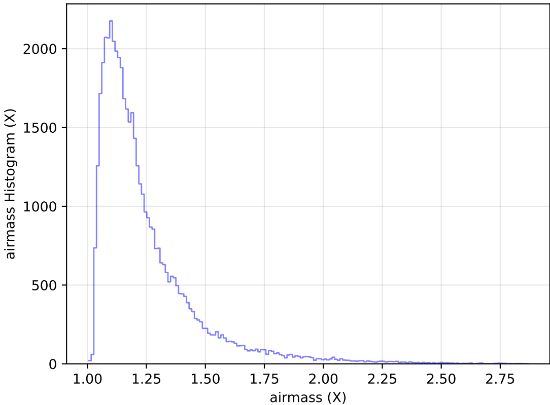
too_elab_r16_d2_ugrizy_v3.4_10yrs Yr 1 y band: airmass Histogram
