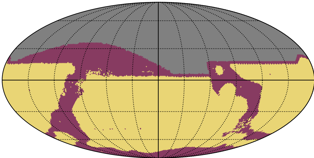
too_elab_r16_d2_ugrizy_v3.4_10yrs All sky: RapidRevisits
