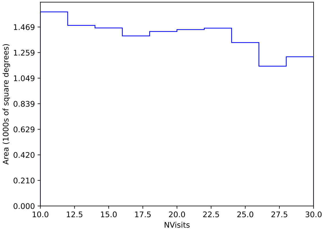
too_elab_r16_d2_ugrizy_v3.4_10yrs Yr 3-4 y band: NVisits
