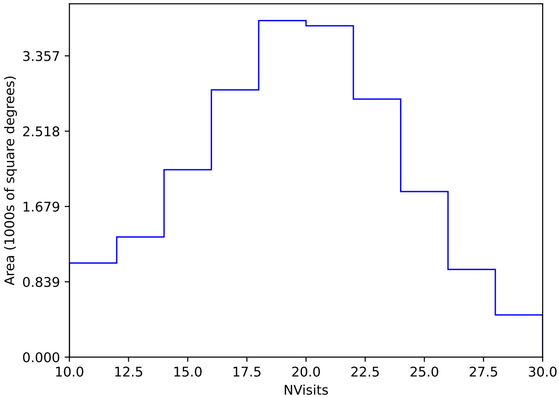
too_elab_r16_d2_ugrizy_v3.4_10yrs Yr 1 y band: NVisits
