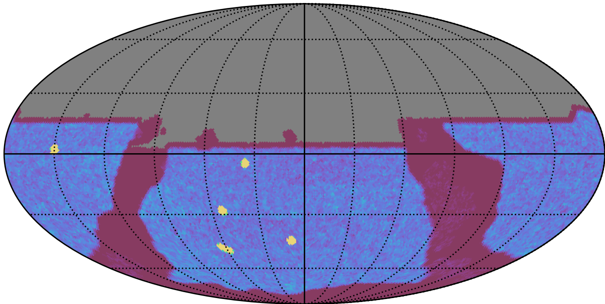
too_elab_r16_d2_ugrizy_v3.4_10yrs All sky y band: NVisits
