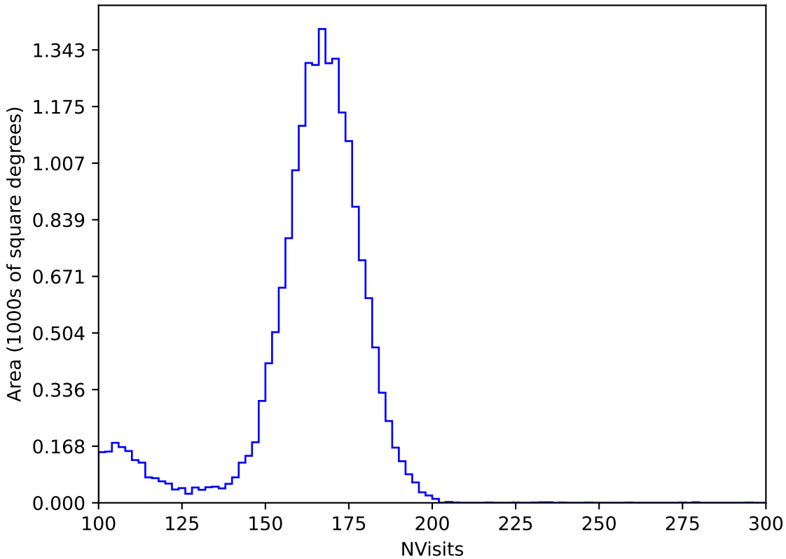
too_elab_r16_d2_ugrizy_v3.4_10yrs All sky y band: NVisits
