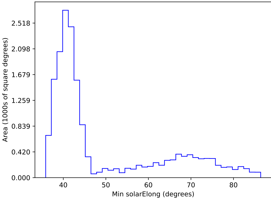
too_elab_r16_d2_ugrizy_v3.4_10yrs WFD z band: Min solarElong
