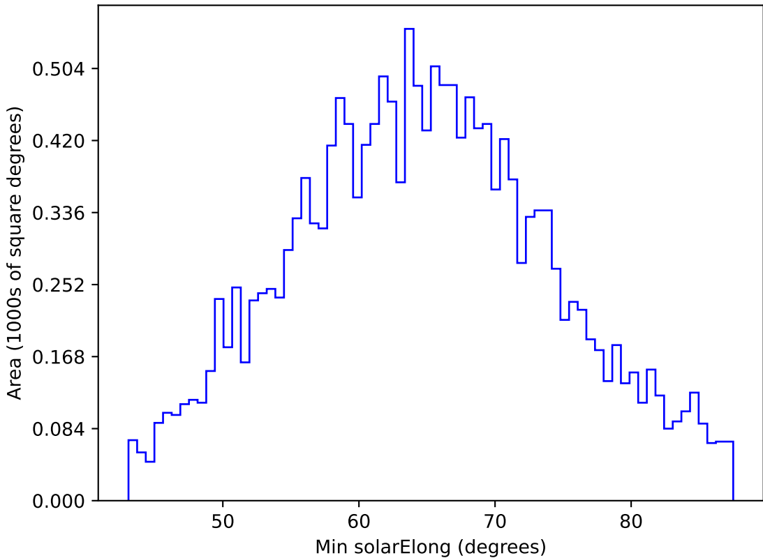
too_elab_r16_d2_ugrizy_v3.4_10yrs WFD y band: Min solarElong
