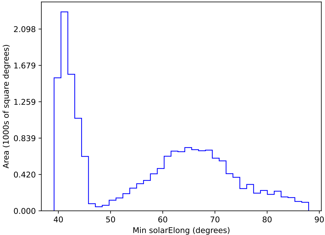
too_elab_r16_d2_ugrizy_v3.4_10yrs WFD r band: Min solarElong
