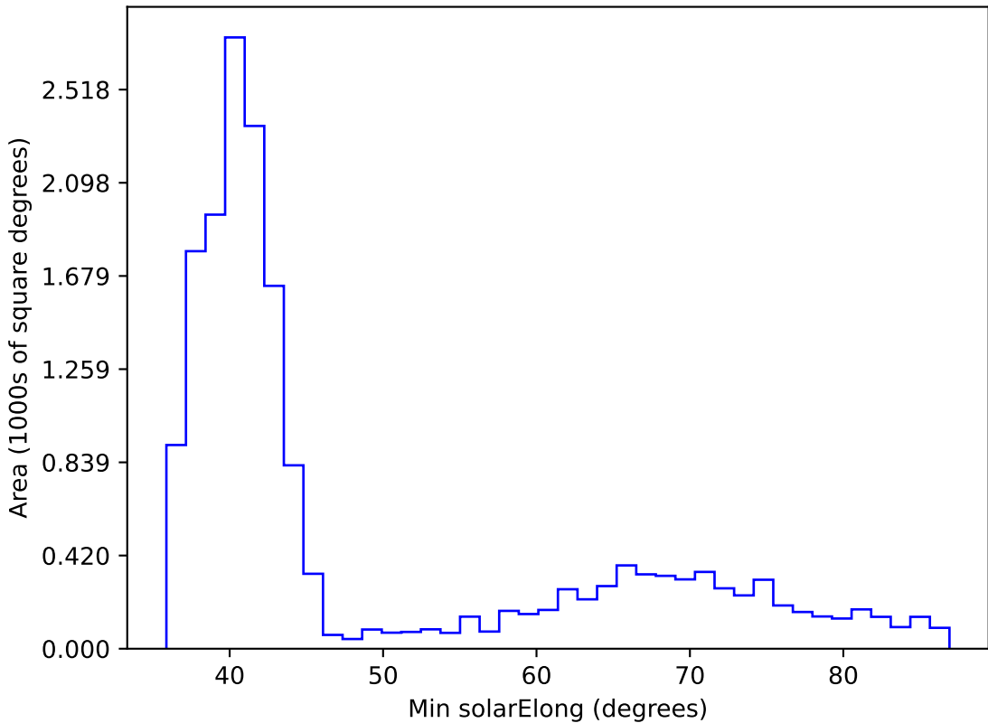
too_elab_r16_d2_ugrizy_v3.4_10yrs WFD i band: Min solarElong
