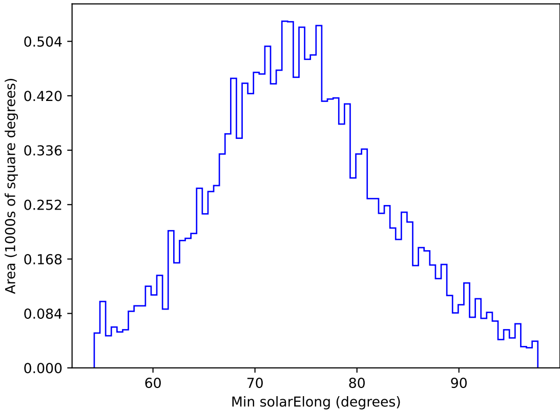
too_elab_r16_d2_ugrizy_v3.4_10yrs WFD g band: Min solarElong
