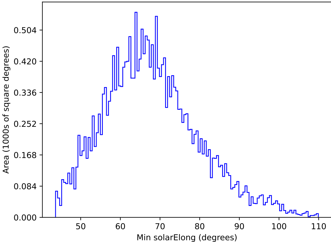
too_elab_r16_d2_ugrizy_v3.4_10yrs All sky y band: Min solarElong
