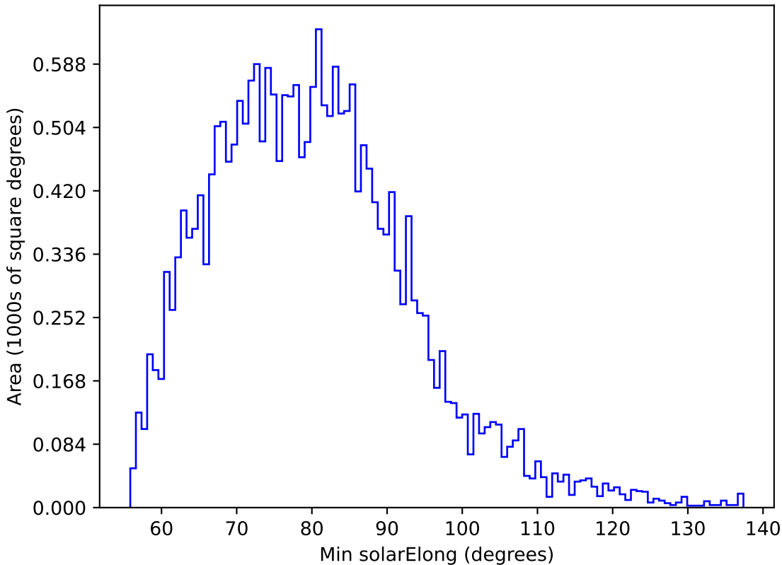
too_elab_r16_d2_ugrizy_v3.4_10yrs All sky u band: Min solarElong
