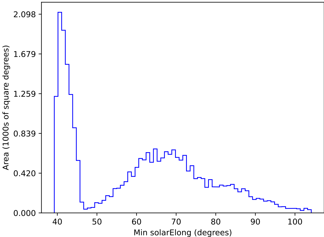
too_elab_r16_d2_ugrizy_v3.4_10yrs All sky r band: Min solarElong
