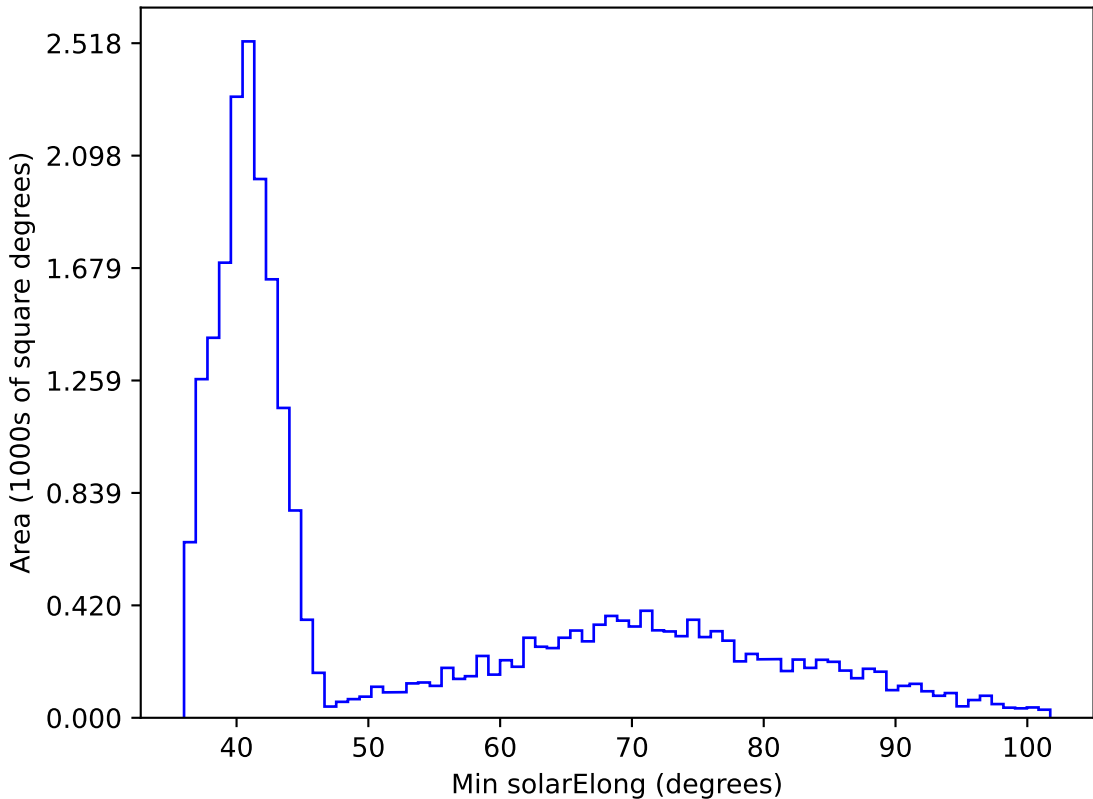
too_elab_r16_d2_ugrizy_v3.4_10yrs All sky i band: Min solarElong
