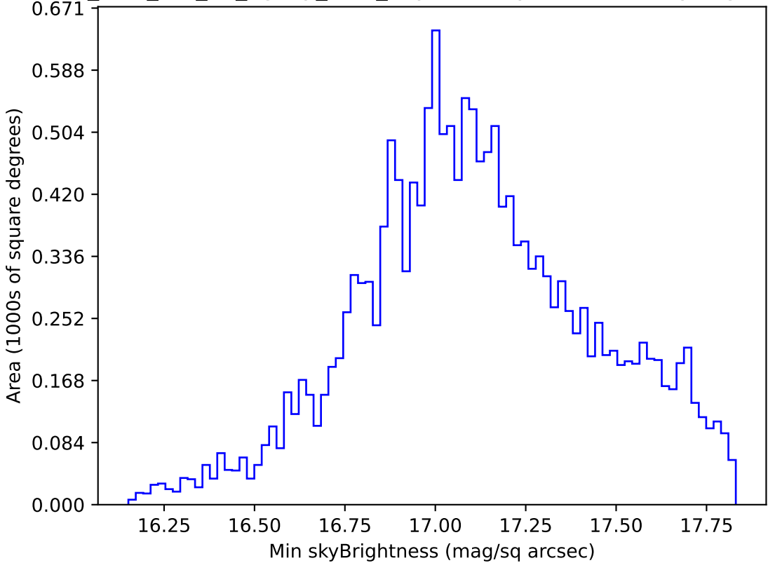
too_elab_r16_d2_ugrizy_v3.4_10yrs WFD y band: Min skyBrightness
