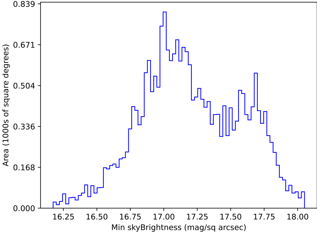
too_elab_r16_d2_ugrizy_v3.4_10yrs All sky y band: Min skyBrightness
