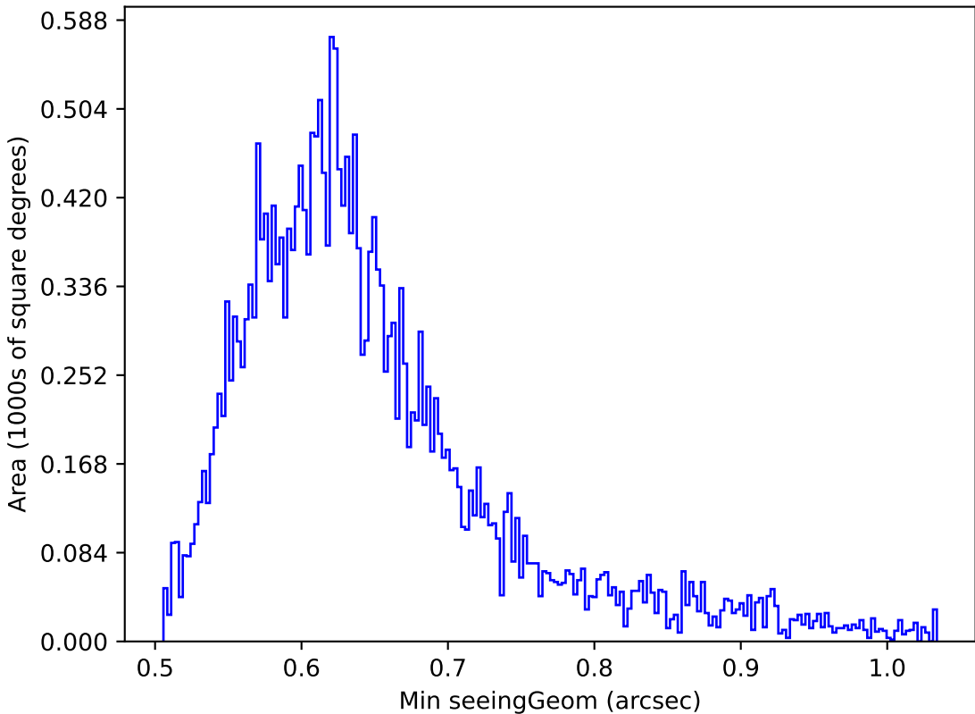
too_elab_r16_d2_ugrizy_v3.4_10yrs Yr 1 z band: Min seeingGeom
