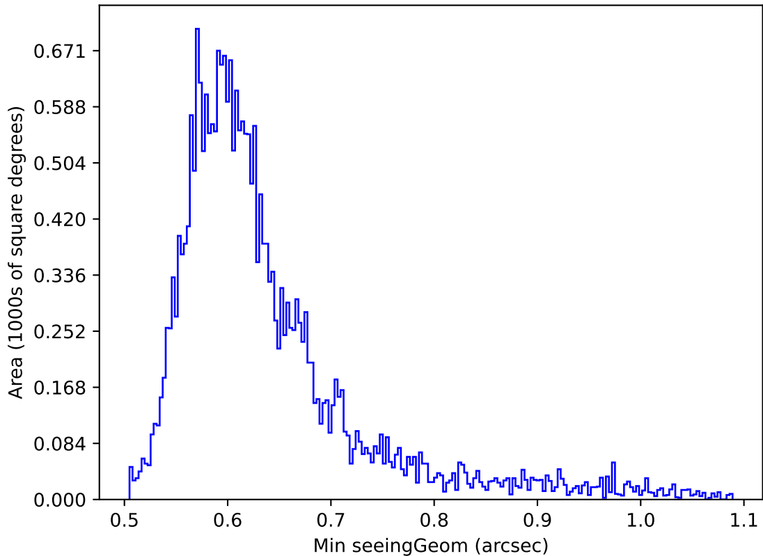
too_elab_r16_d2_ugrizy_v3.4_10yrs Yr 1 i band: Min seeingGeom
