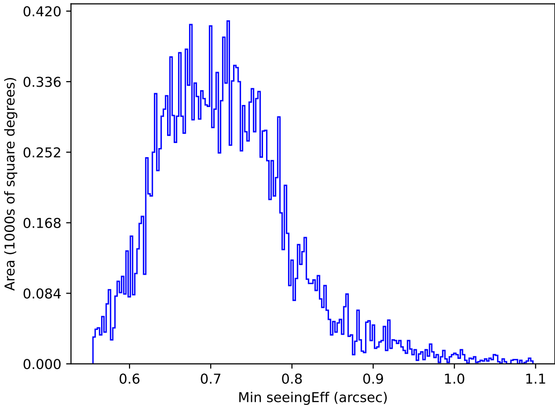
too_elab_r16_d2_ugrizy_v3.4_10yrs Yr 1 y band: Min seeingEff
