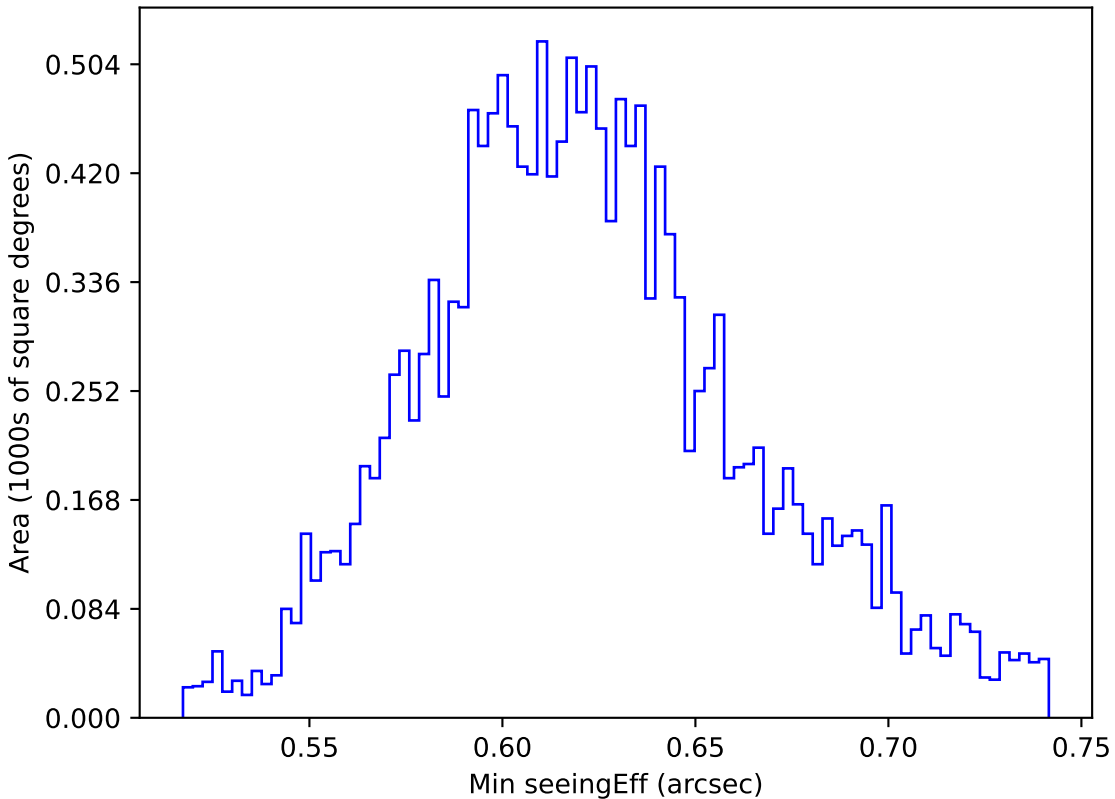
too_elab_r16_d2_ugrizy_v3.4_10yrs WFD y band: Min seeingEff
