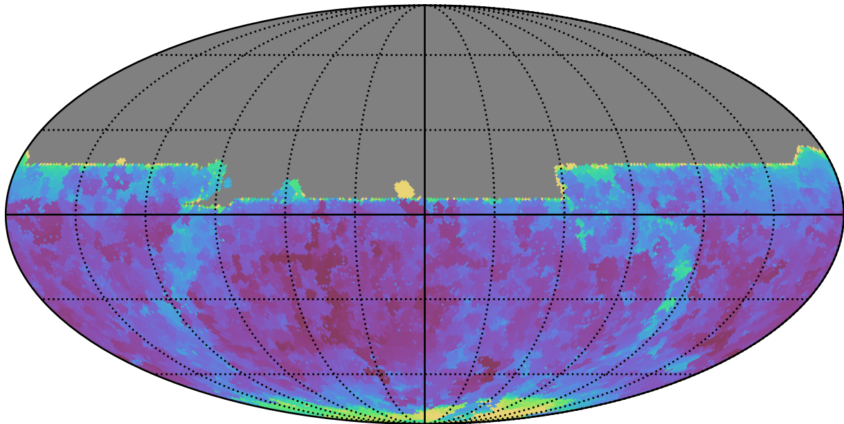
too_elab_r16_d2_ugrizy_v3.4_10yrs All sky y band: Min seeingEff
