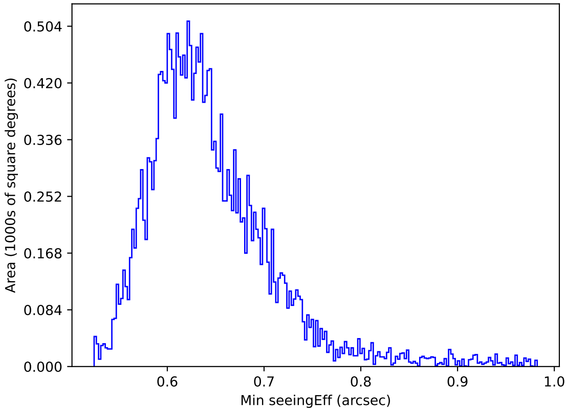
too_elab_r16_d2_ugrizy_v3.4_10yrs All sky y band: Min seeingEff
