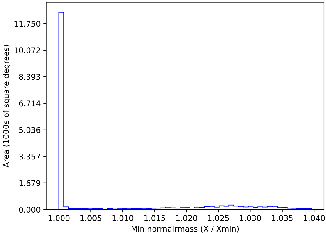
too_elab_r16_d2_ugrizy_v3.4_10yrs WFD y band: Min normairmass
