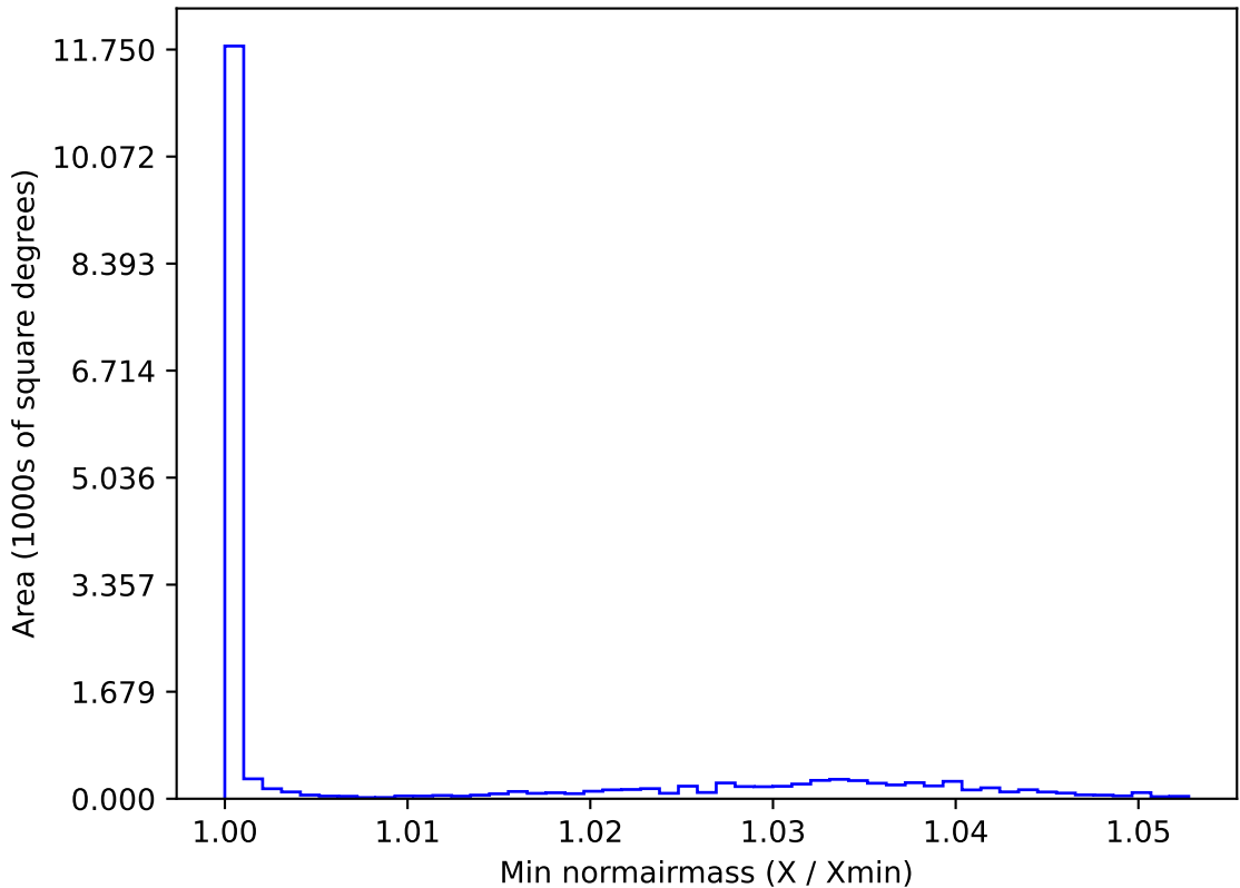
too_elab_r16_d2_ugrizy_v3.4_10yrs WFD u band: Min normairmass
