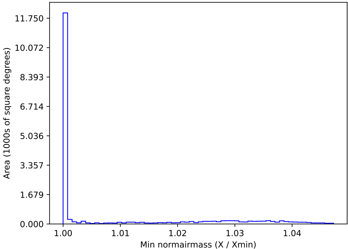
too_elab_r16_d2_ugrizy_v3.4_10yrs WFD g band: Min normairmass
