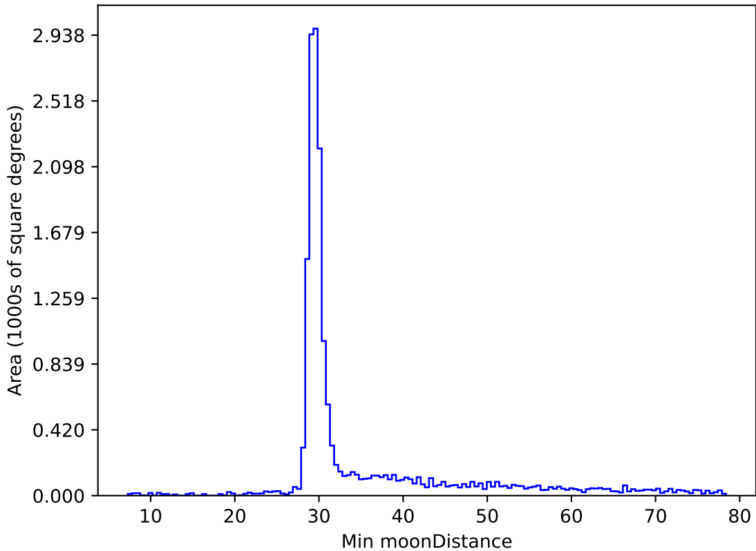
too_elab_r16_d2_ugrizy_v3.4_10yrs WFD y band: Min moonDistance
