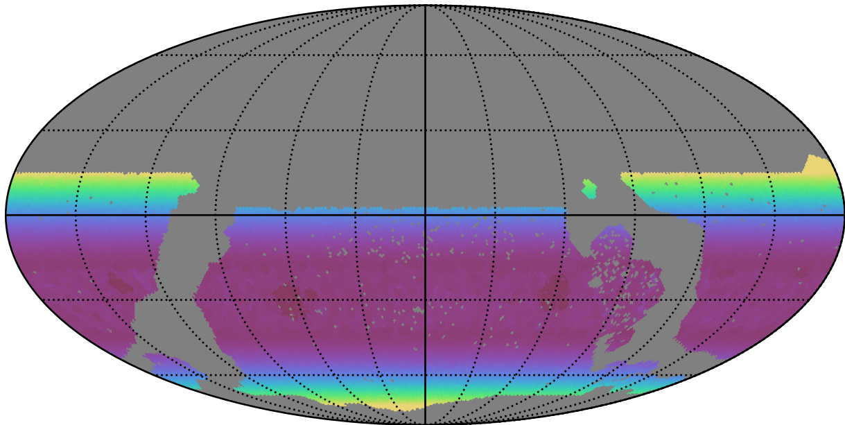
too_elab_r16_d2_ugrizy_v3.4_10yrs WFD y band: Min airmass
