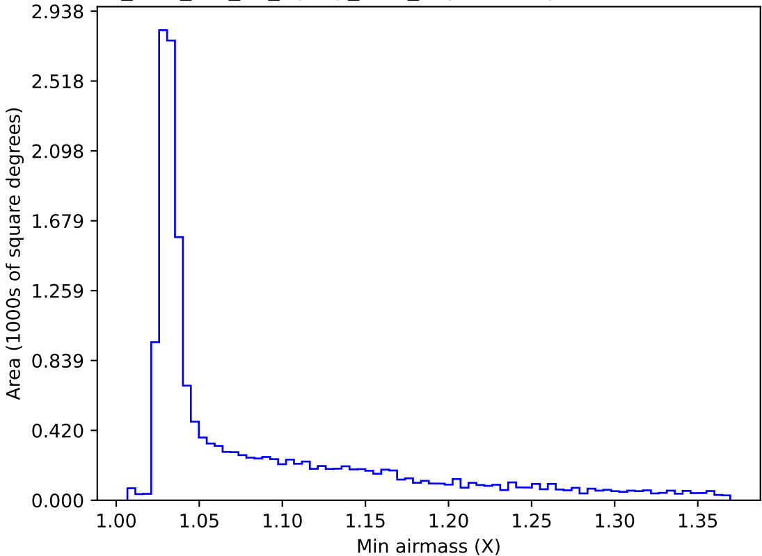
too_elab_r16_d2_ugrizy_v3.4_10yrs WFD y band: Min airmass
