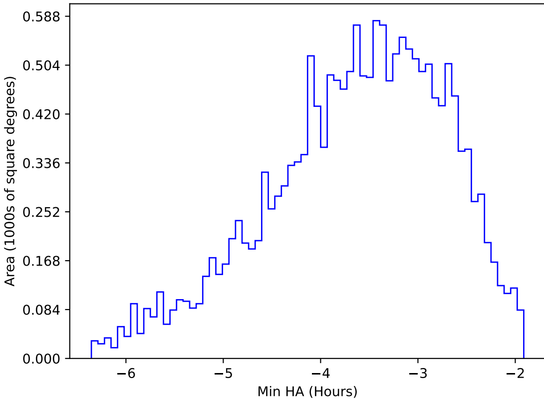
too_elab_r16_d2_ugrizy_v3.4_10yrs WFD y band: Min HA
