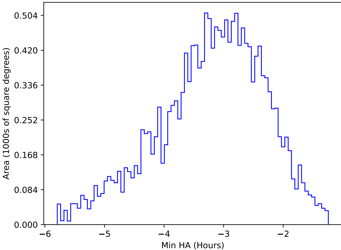
too_elab_r16_d2_ugrizy_v3.4_10yrs WFD u band: Min HA
