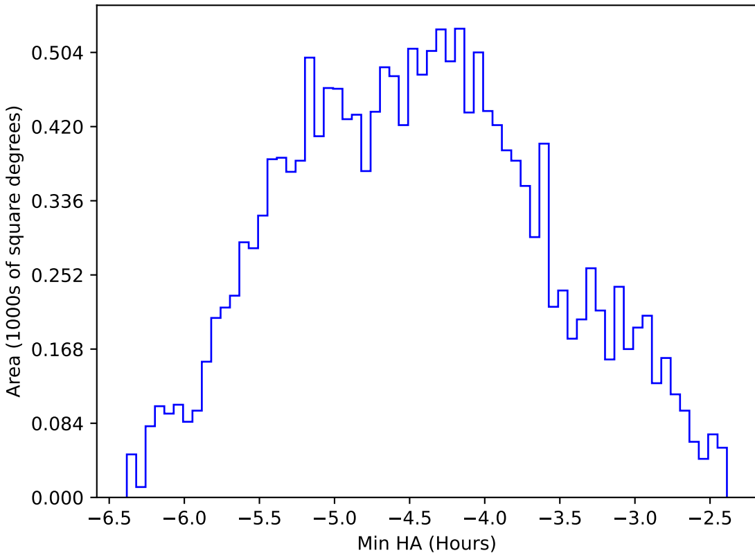
too_elab_r16_d2_ugrizy_v3.4_10yrs WFD r band: Min HA
