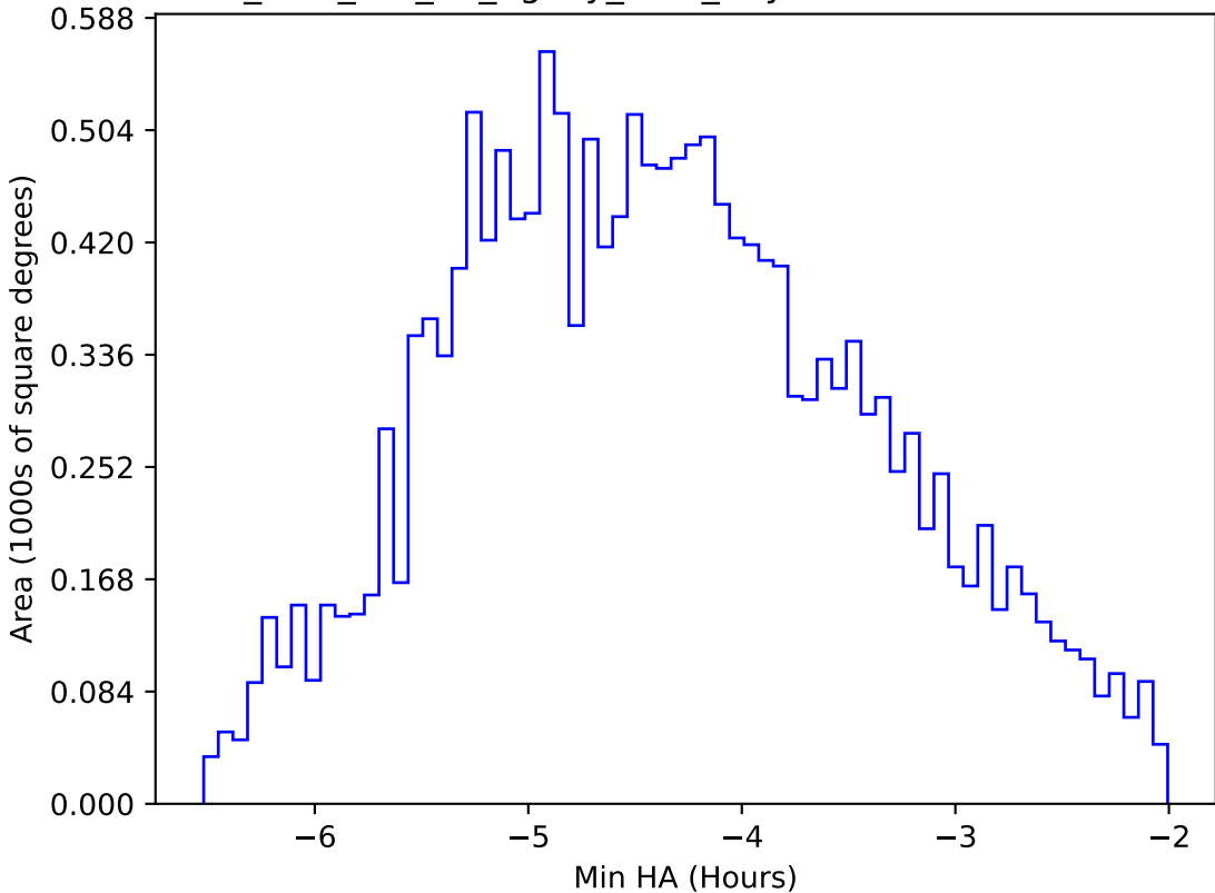
too_elab_r16_d2_ugrizy_v3.4_10yrs WFD i band: Min HA
