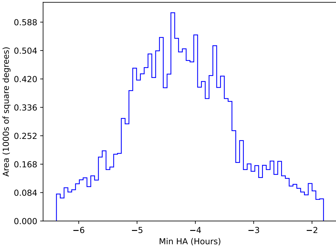
too_elab_r16_d2_ugrizy_v3.4_10yrs WFD g band: Min HA
