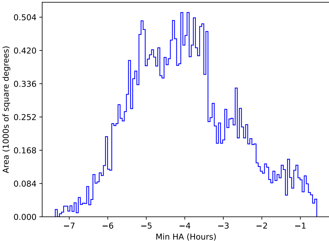
too_elab_r16_d2_ugrizy_v3.4_10yrs All sky z band: Min HA
