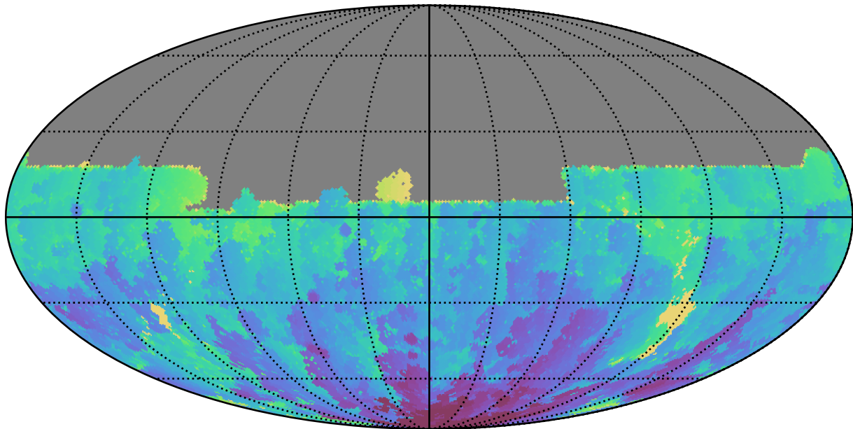
too_elab_r16_d2_ugrizy_v3.4_10yrs All sky u band: Min HA
