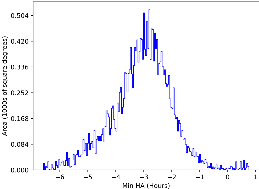
too_elab_r16_d2_ugrizy_v3.4_10yrs All sky u band: Min HA
