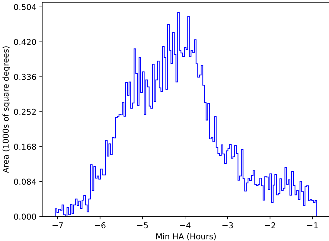
too_elab_r16_d2_ugrizy_v3.4_10yrs All sky r band: Min HA
