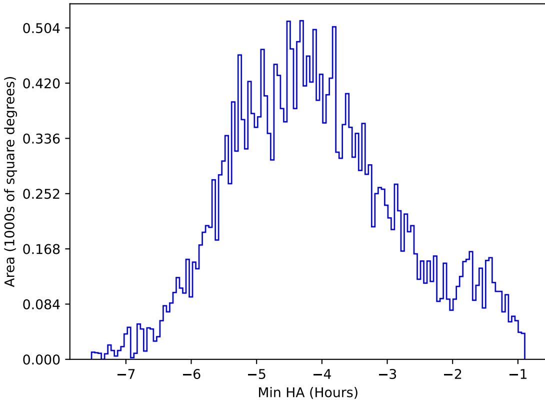
too_elab_r16_d2_ugrizy_v3.4_10yrs All sky i band: Min HA
