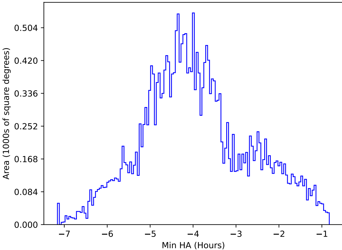
too_elab_r16_d2_ugrizy_v3.4_10yrs All sky g band: Min HA
