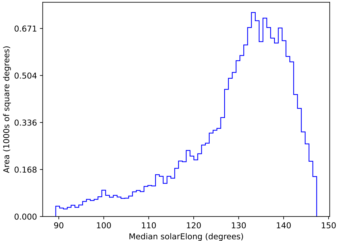
too_elab_r16_d2_ugrizy_v3.4_10yrs WFD y band: Median solarElong
