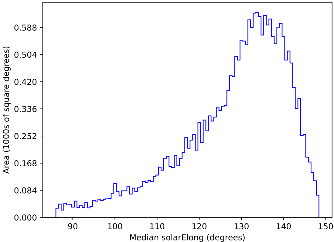
too_elab_r16_d2_ugrizy_v3.4_10yrs All sky y band: Median solarElong
