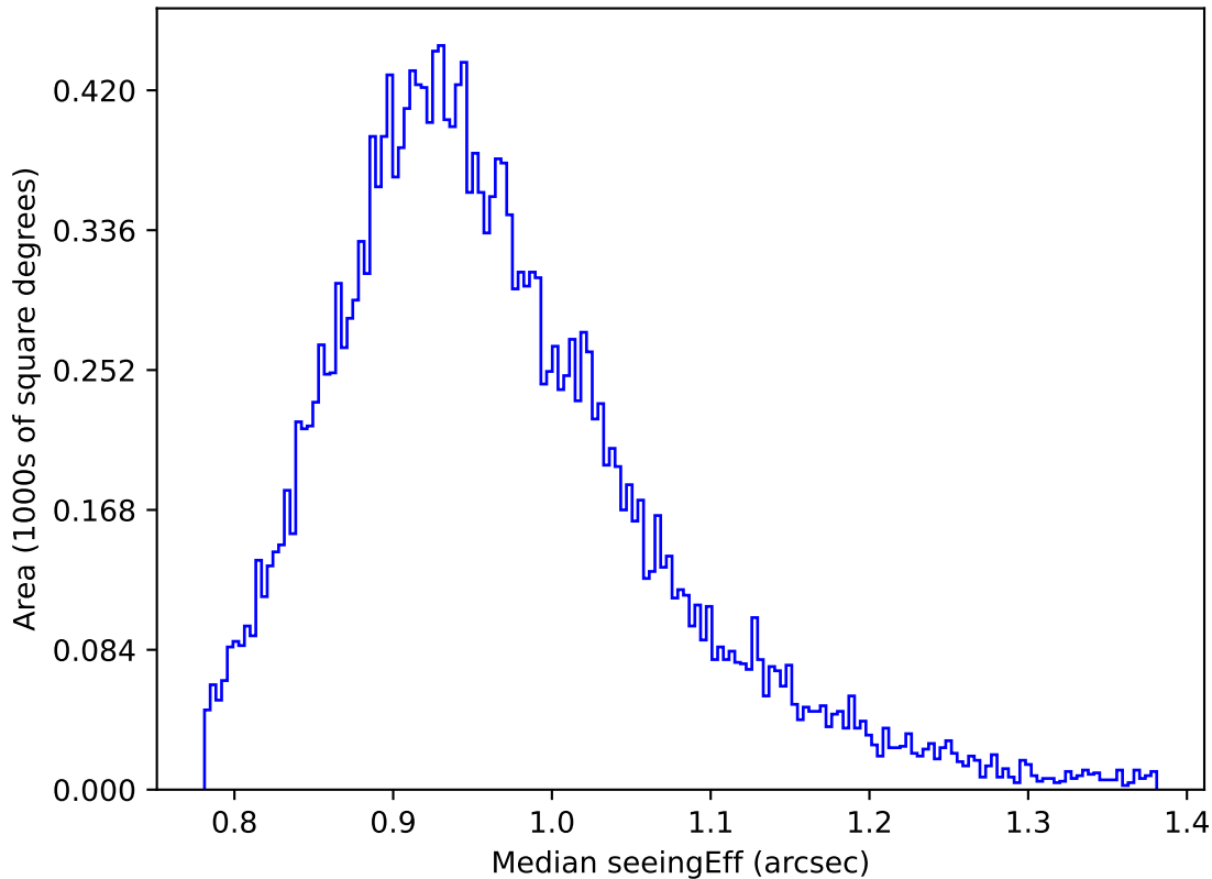
too_elab_r16_d2_ugrizy_v3.4_10yrs Yr 1 y band: Median seeingEff
