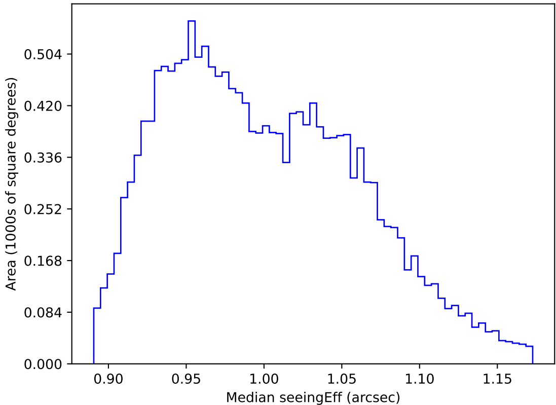
too_elab_r16_d2_ugrizy_v3.4_10yrs WFD y band: Median seeingEff
