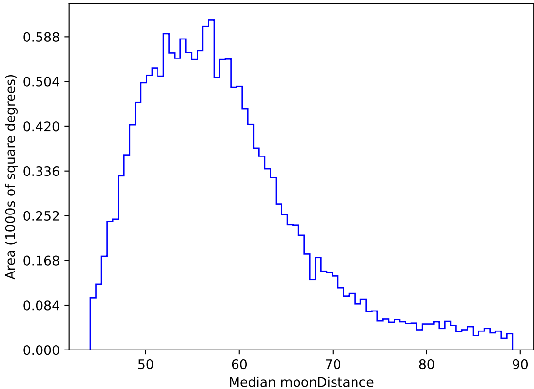
too_elab_r16_d2_ugrizy_v3.4_10yrs WFD y band: Median moonDistance
