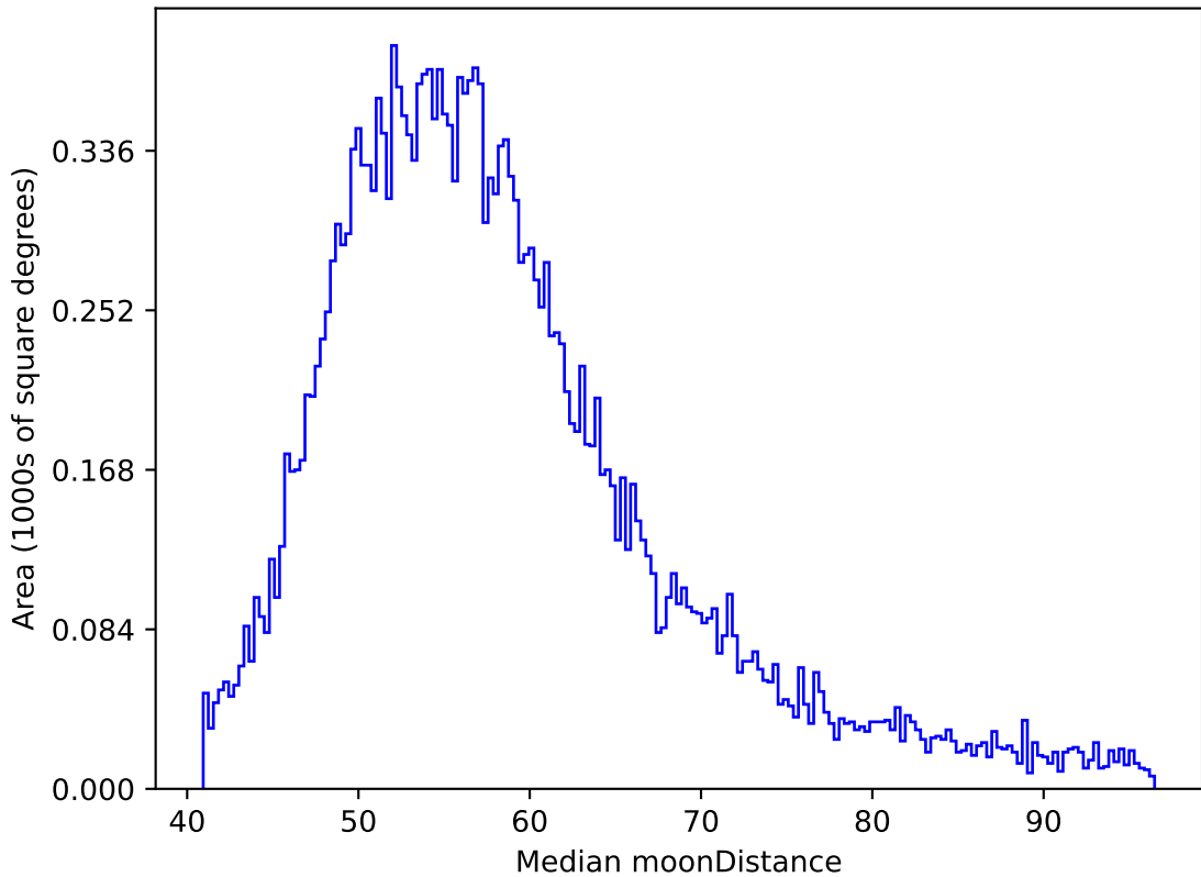
too_elab_r16_d2_ugrizy_v3.4_10yrs All sky y band: Median moonDistance
