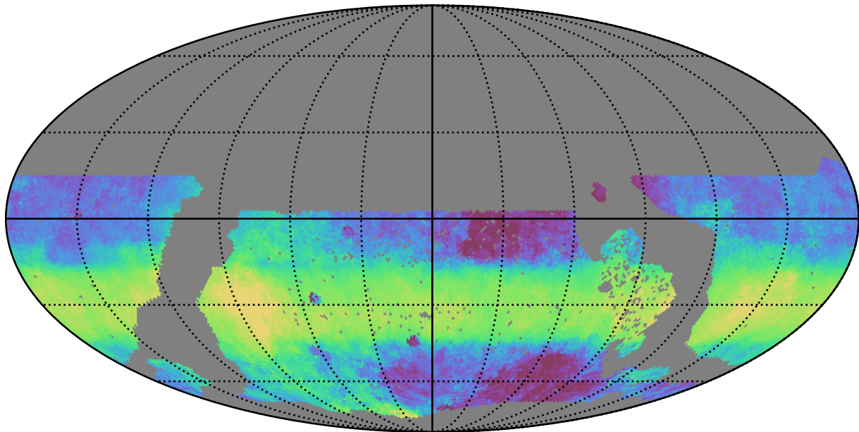
too_elab_r16_d2_ugrizy_v3.4_10yrs WFD y band: Median HA
