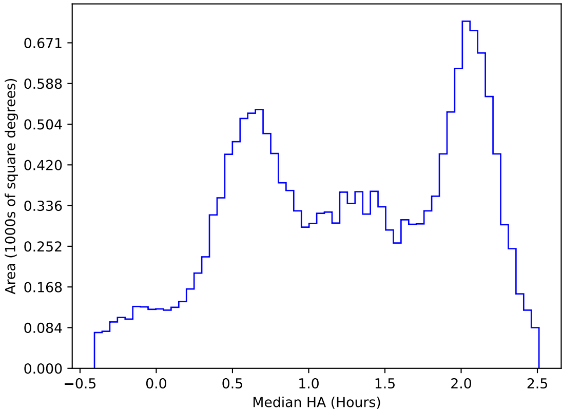
too_elab_r16_d2_ugrizy_v3.4_10yrs WFD y band: Median HA
