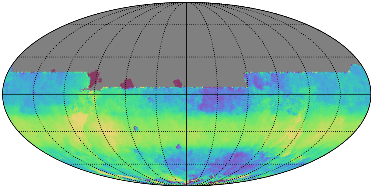
too_elab_r16_d2_ugrizy_v3.4_10yrs All sky y band: Median HA
